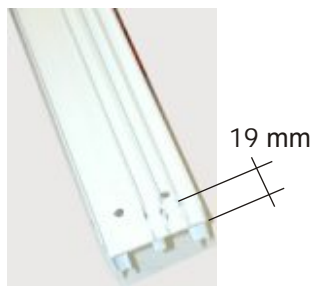
нажня часть
